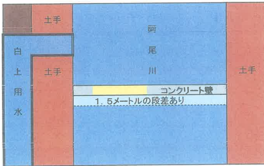
取水口上面図
